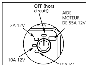
Figure 3 – Contrôles du chargeur
